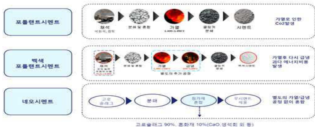
<포틀랜드 시멘트, 백색시멘트, 네오시멘트 제조공정 비교>
